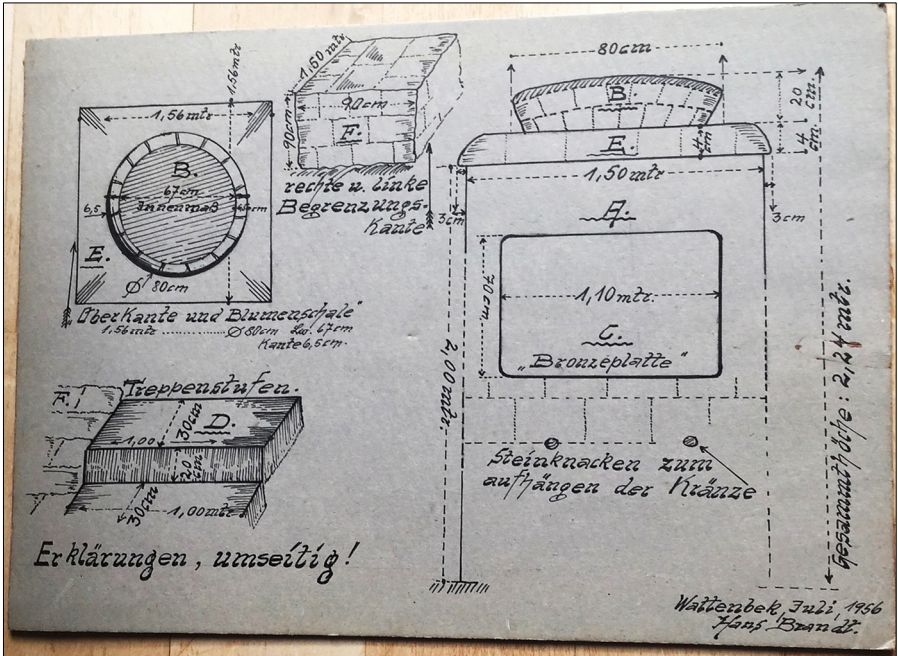
Die technischen Daten des Entwurfs des Ehrenmals
